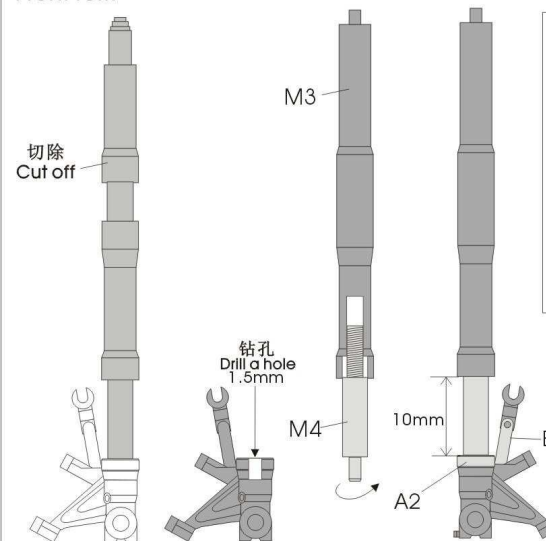
前叉 Front fork
