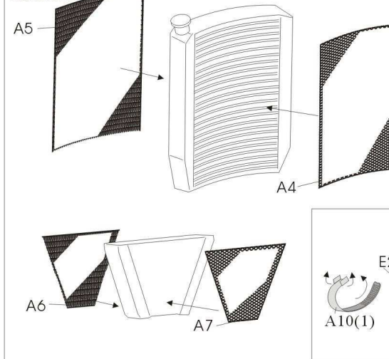
散熱器 Radiator
