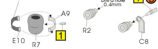
黑色膠貼 Black band
