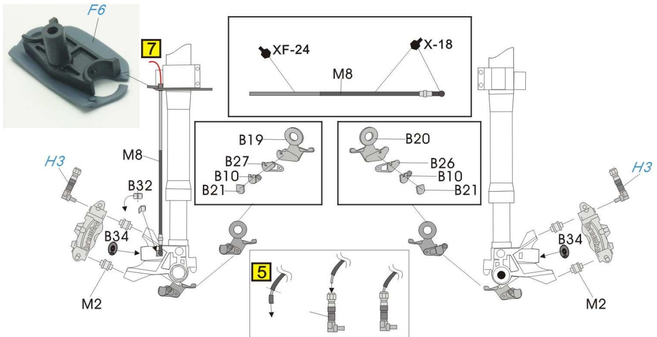
Front fork 前叉
